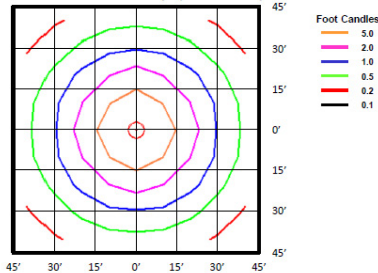
CPLED-13-4K-###-UNV (12,516 Lumens)
