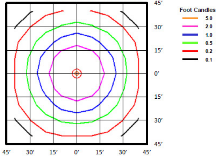
CPLED-7-4K-###-UNV (7,002 Lumens)
