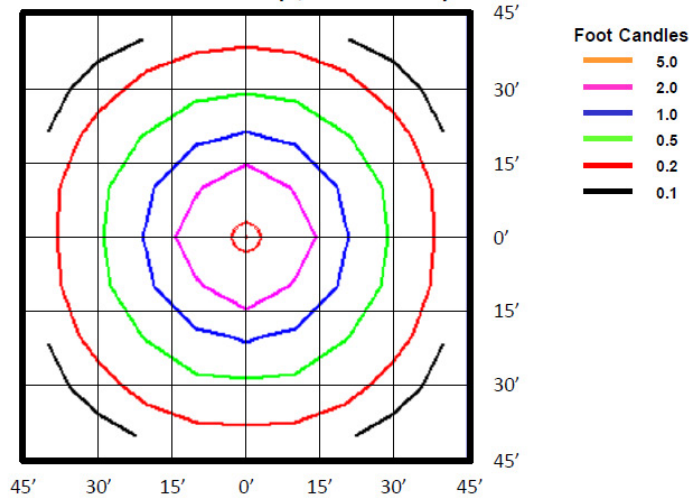
CPLED-5-4K-###-UNV (4,943 Lumens)
