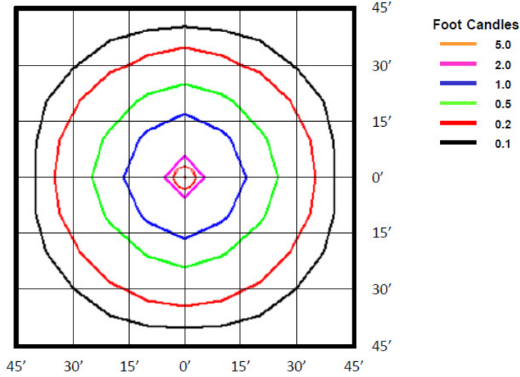
CPLED-3-4K-###-UNV (3,137 Lumens)
